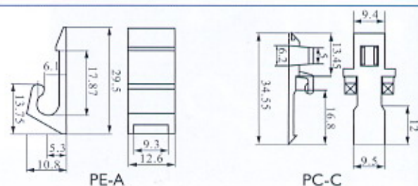
方形卡扣 PE PC Clip
